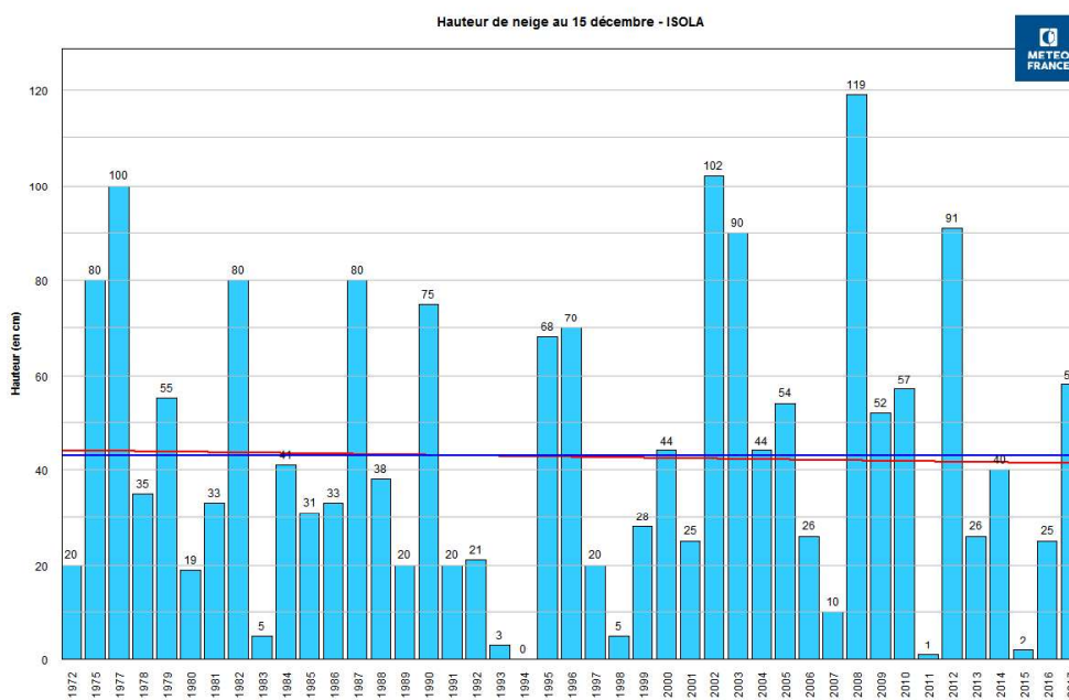
Figure 3. Tendances de la hauteur de neige au 15 décembre à Isola entre 1972 et 2017. La moyenne est en bleu, la courbe d'ajustement en rouge
