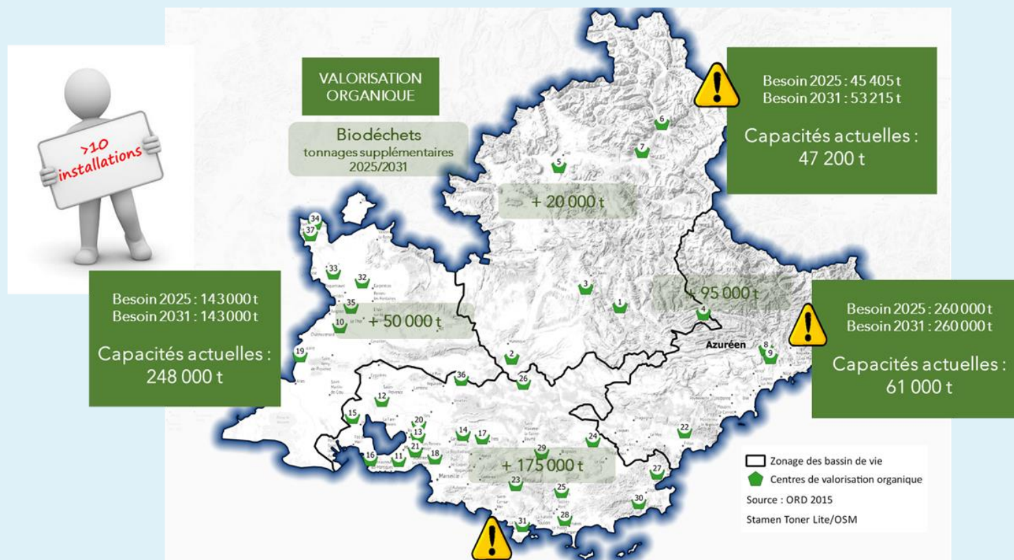
Figure 9 : Installations qu'il apparaît nécessaire de créer, d'adapter ou de fermer – Unités de valorisation organique
