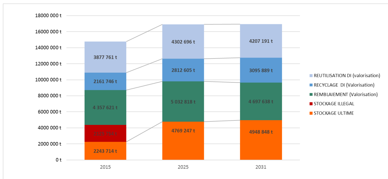
Figure 5 : Evolution régionale des productions de déchets inertes à traiter par filière aux échéances 2025 et 2031
