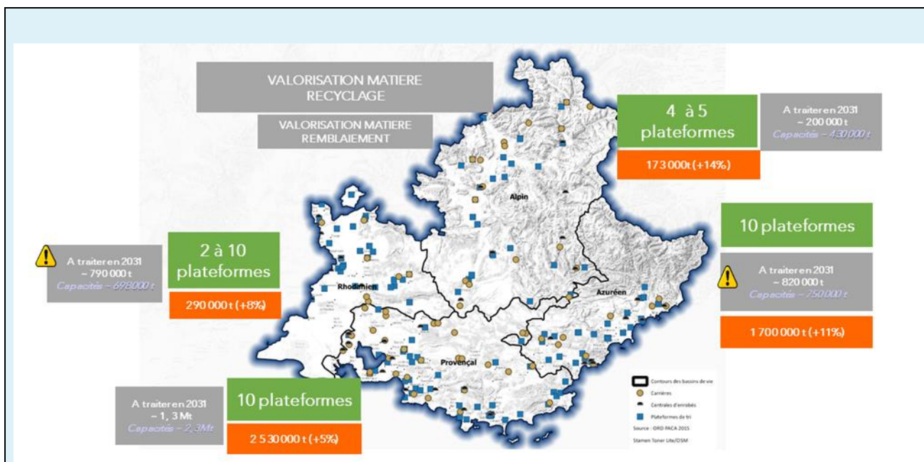
Figure 16 : Plateformes de recyclage qu'il apparaît nécessaire de créer, d'adapter ou de fermer afin d'atteindre les objectifs en cohérence avec les principes de proximité et d'autosuffisance, adaptés aux bassins de vie.
